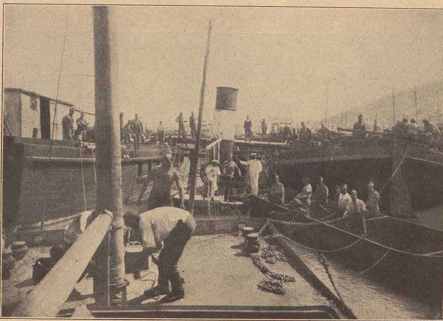
Bergung des versenkten italienischen Dampfers „Neptun“ durch Linzer Pioniere.
