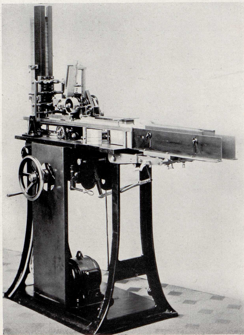
Abb. 108. Hofherr-Signettiermaschine, Modell EA
