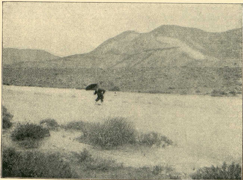
Abb. 10. Regenfluten in einem Trockental.
