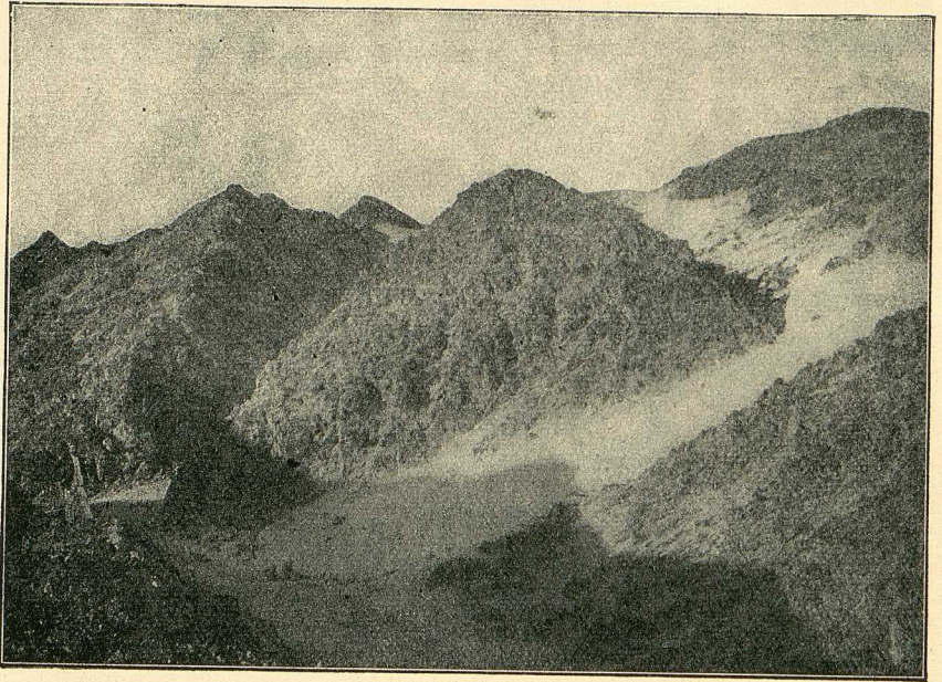
Abb. 7. Sandfelder im Granit der südlichen Sinaiwüste. Phot. Natterer.
