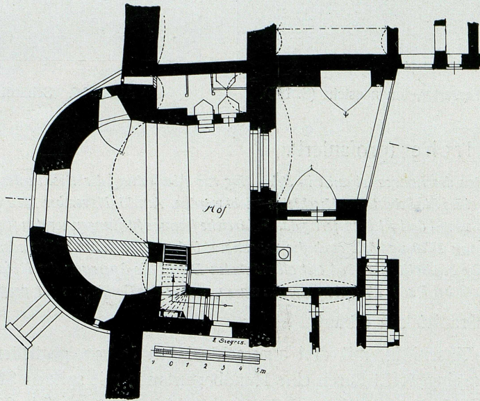
Abb. 214. Schärding, Wassertor, Grundriß 1: 300 (S. 195).
