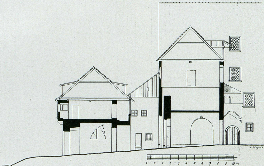
Abb. 213. Schärding, Wassertor, Längenschnitt 1: 300 (S. 195).
