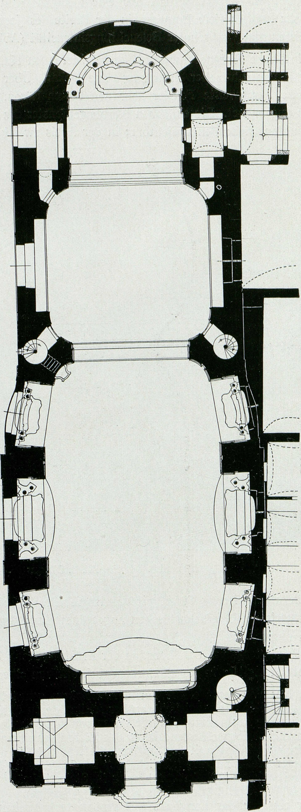
Abb. 12. Engelszell, Klosterkirche, Grundriß 1 : 300 (S. 14).
